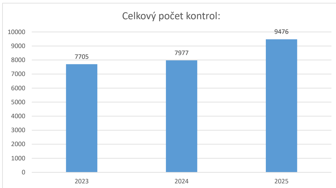
Text v obrázku: Celkový počet kontrol
